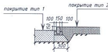
Сечение а-а
